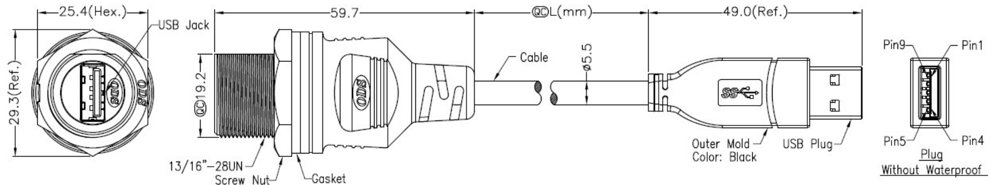
寸法図
