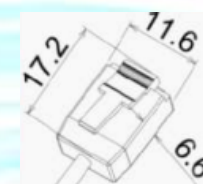
コネクタ寸法図
